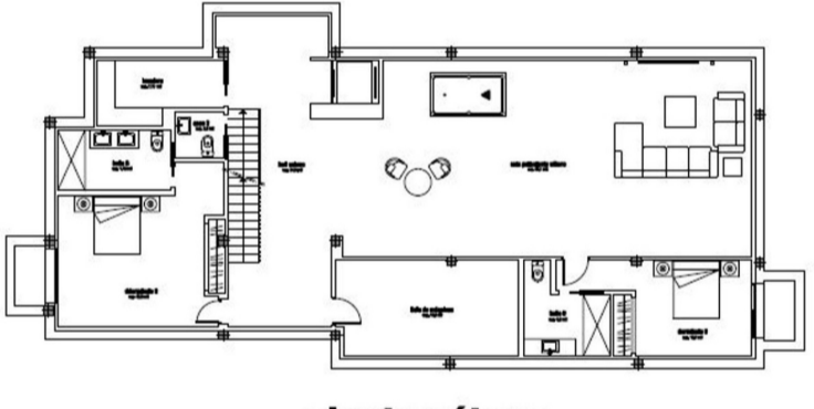
planta sótano
